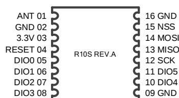
图 4 引脚排序
