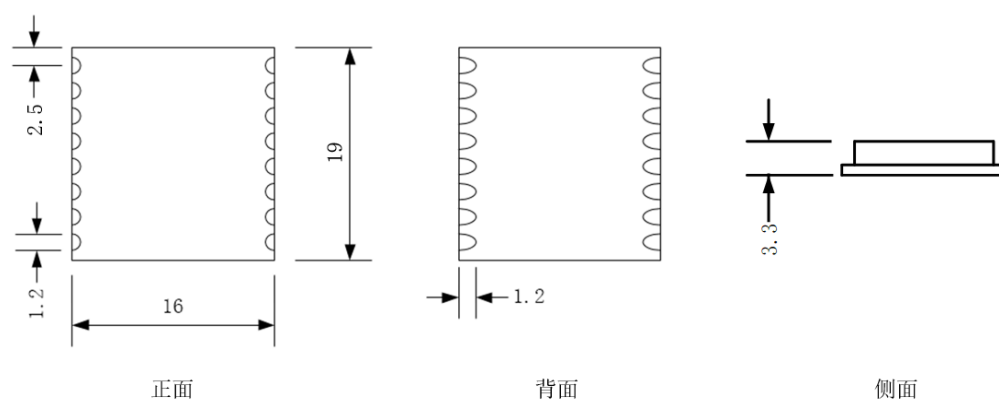
图 6 R10S 机械尺寸及封装
